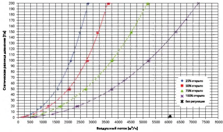
График сопротивления Стальная вентиляционная плита 600x600, перфорация 50 %
